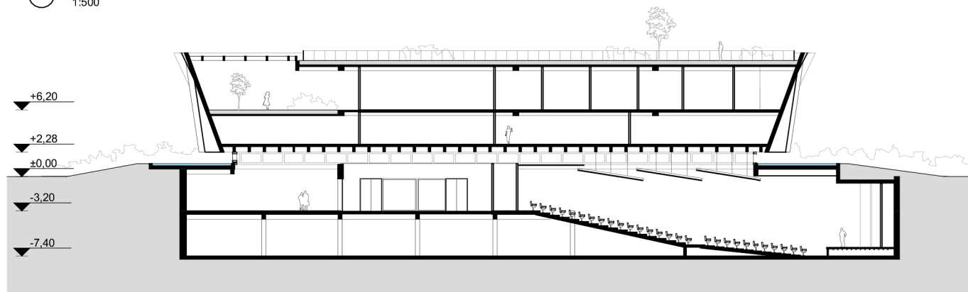
3 CORTE AA ESCALA: 1:500
