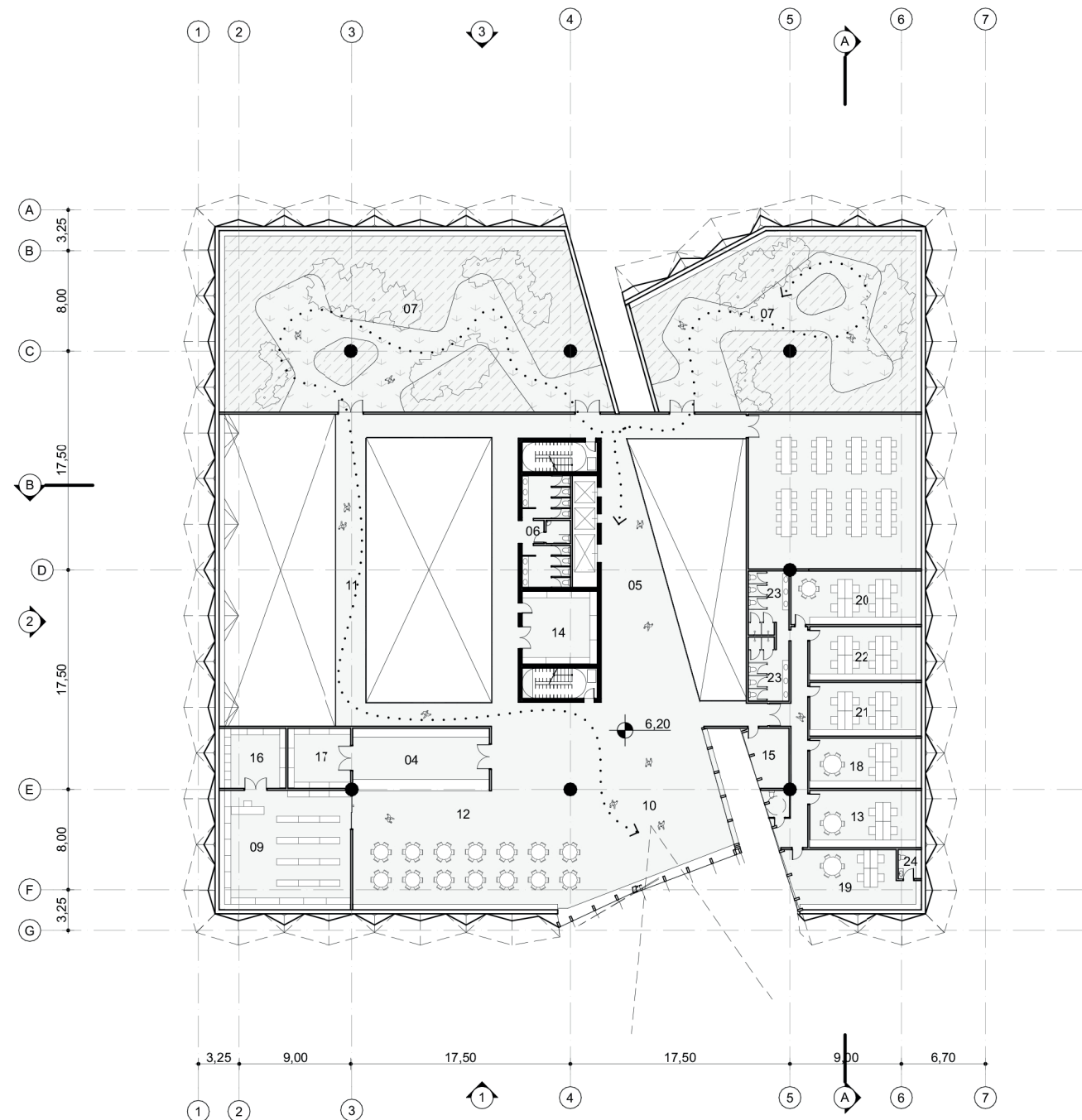
1 PLANTA 2º ANDAR 1:500
