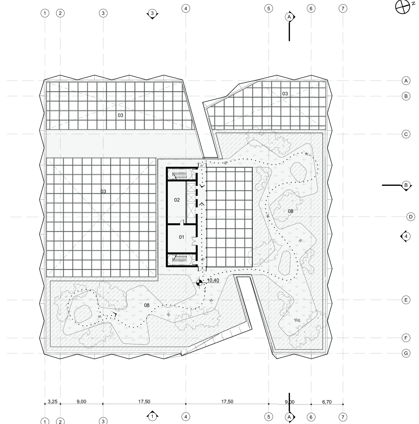
2 PLANTA ACESSO COB. 1:500
