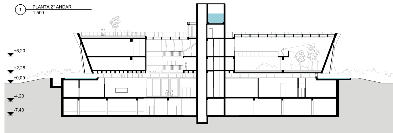
3 CORTE BB ESCALA: 1:500
