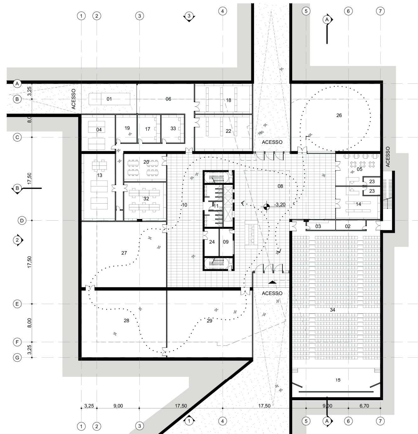
1 PLANTA NÍVEL DE ACESSO 1:500
