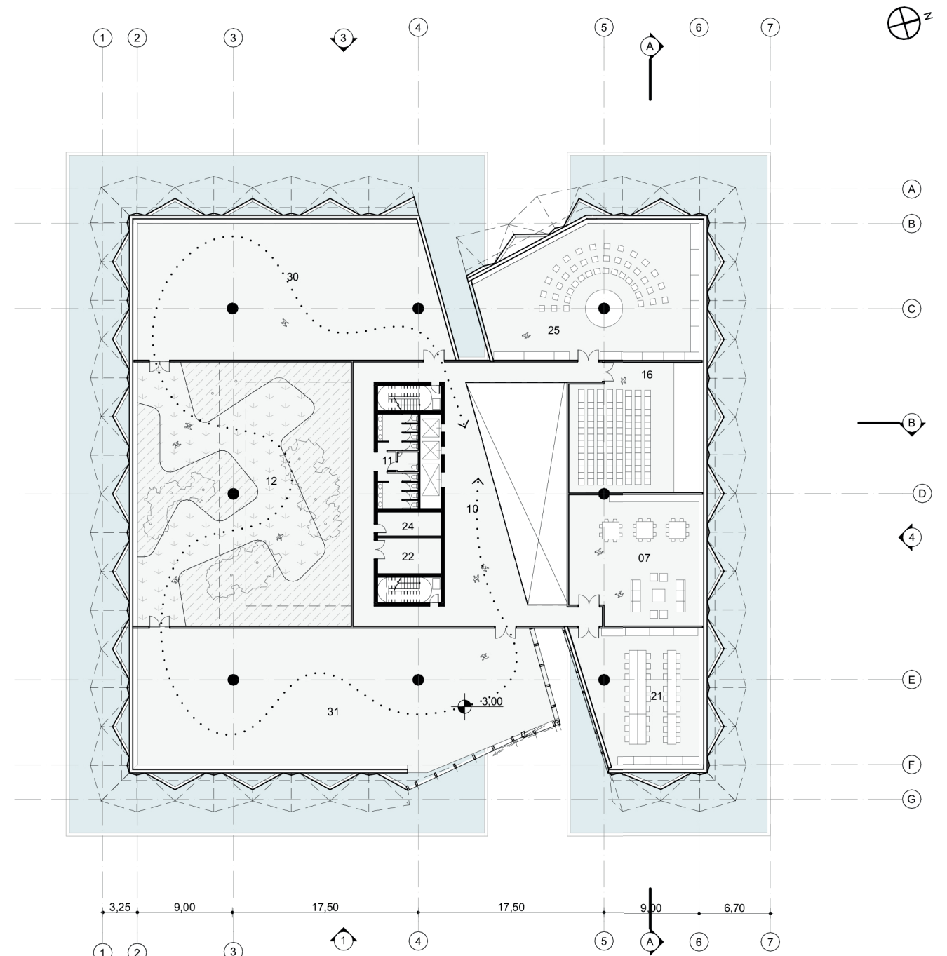
2 PLANTA 1º ANDAR 1:500
