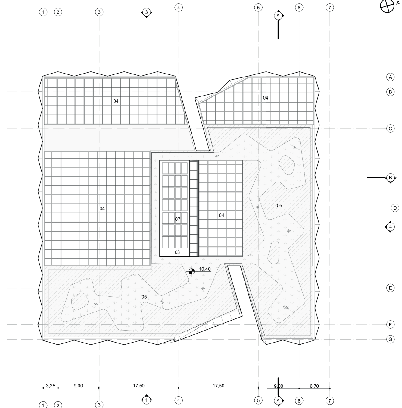
2 PLANTA DE COBERTURA 1:500
