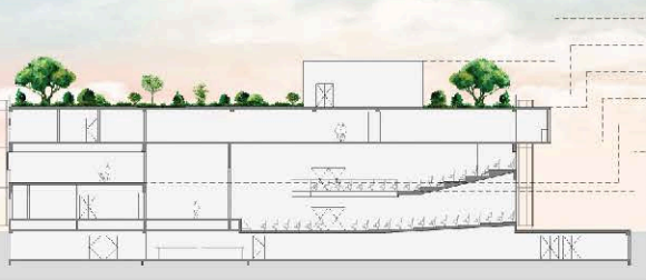
CORTE BB
